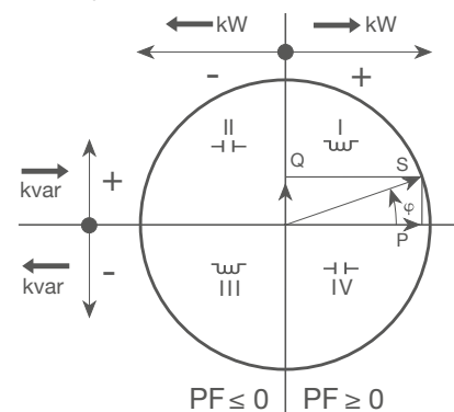
Factor de potência Convenção de acordo com IEC 62053-23
