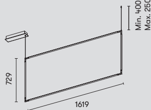
00-8271-05-M1 ■ 100-305V (DALI) 00-8299-05-M1 ■ 176-305V
