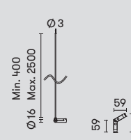
71-8253-05-05 ■ 120° connector - Conector 120° - Connecteur 120°
