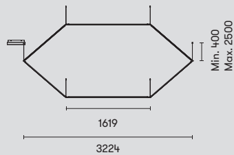
00-8278-05-M1 ■ 90-305V (DALI)
