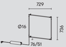
05-8255-05-M1 ■ 90-305V (PWM)
