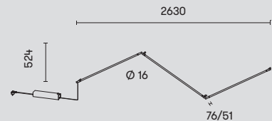
05-8291-05-M1 ■ 90-305V (PWM)
