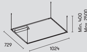
00-8259-05-M1 ■ 100-305V (DALI) 00-8295-05-M1 ■ 176-305V
