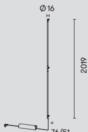
05-8250-05-M1 ■ 90-305V (PWM)
