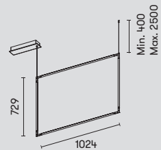
00-8269-05-M1 ■ 100-305V (DALI) 00-8298-05-M1 ■ 176-305V
