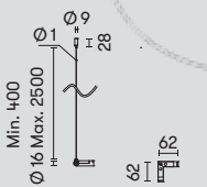
71-8259-05-05 ■ 90° horizontal connector - Conector 90° horizontal - Connecteur 90° horizontal
