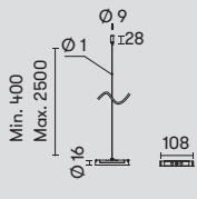
71-8262-05-05 ■ Linear connector - Conector lineal - Connecteur linéaire
