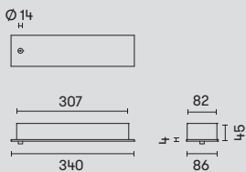
71-8266-05-05 100-305V (DALI) Max. 105W
