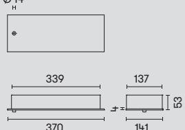
71-8268-05-05 90-305V (DALI) Max. 320W
